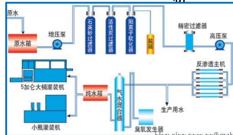
反渗透膜法示意图
